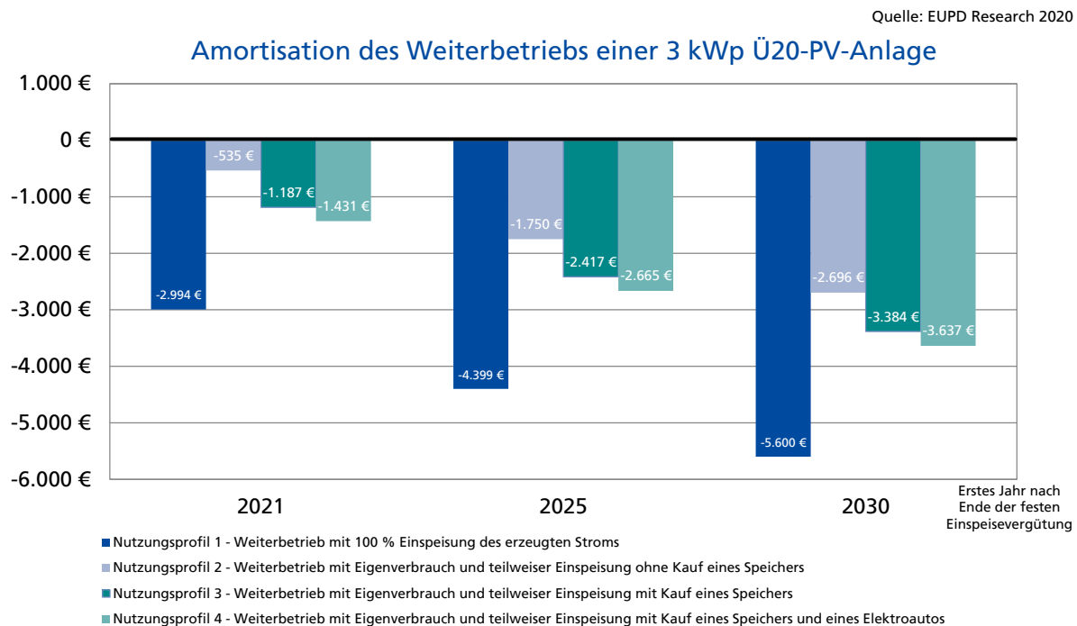
Abbildung 6: Amortisation des Weiterbetriebs einer 3 kWp Ü20-Anlagen für 10 weitere Jahre
