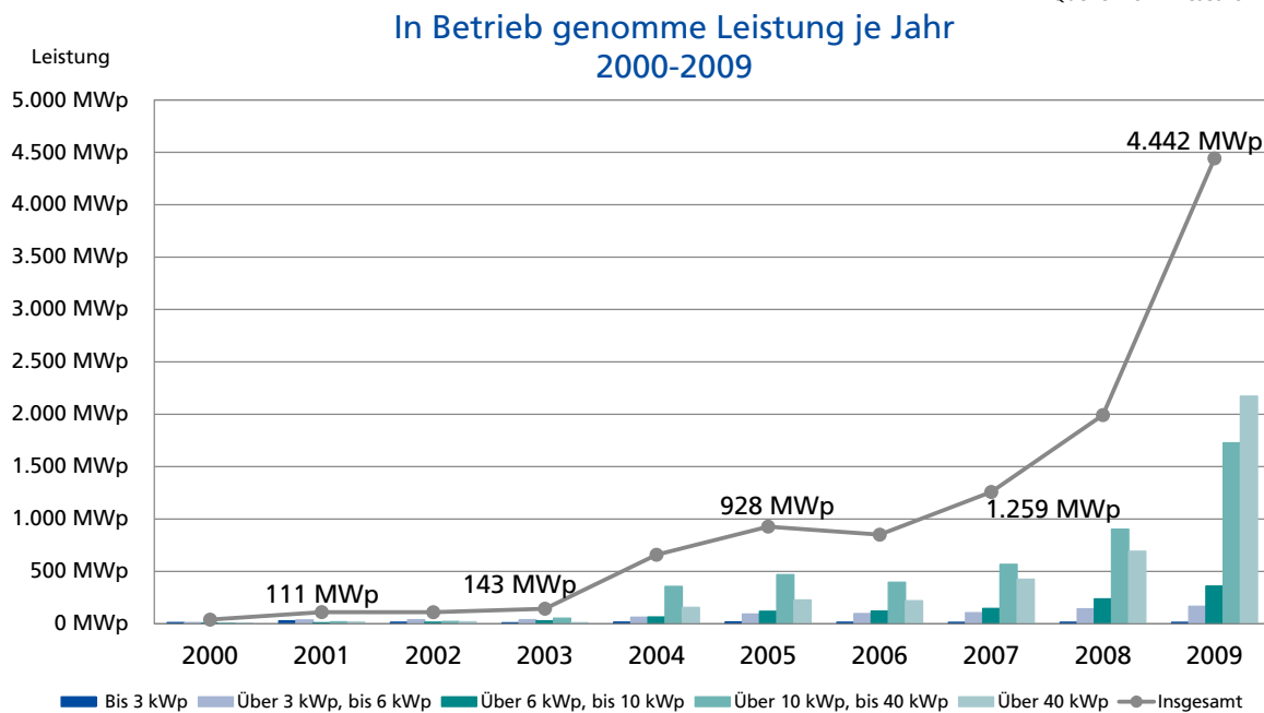
Abbildung 2: In Betrieb genommene Leistung je Jahr nach Größenklassen (2000-2009)
