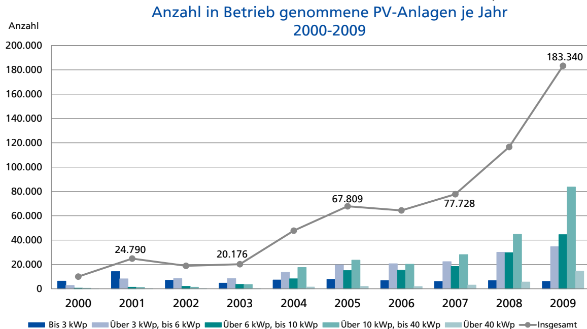
Abbildung 1: Anzahl der in Betrieb genommenen PV-Anlagen je Jahr nach Größenklassen (2000-2009)
